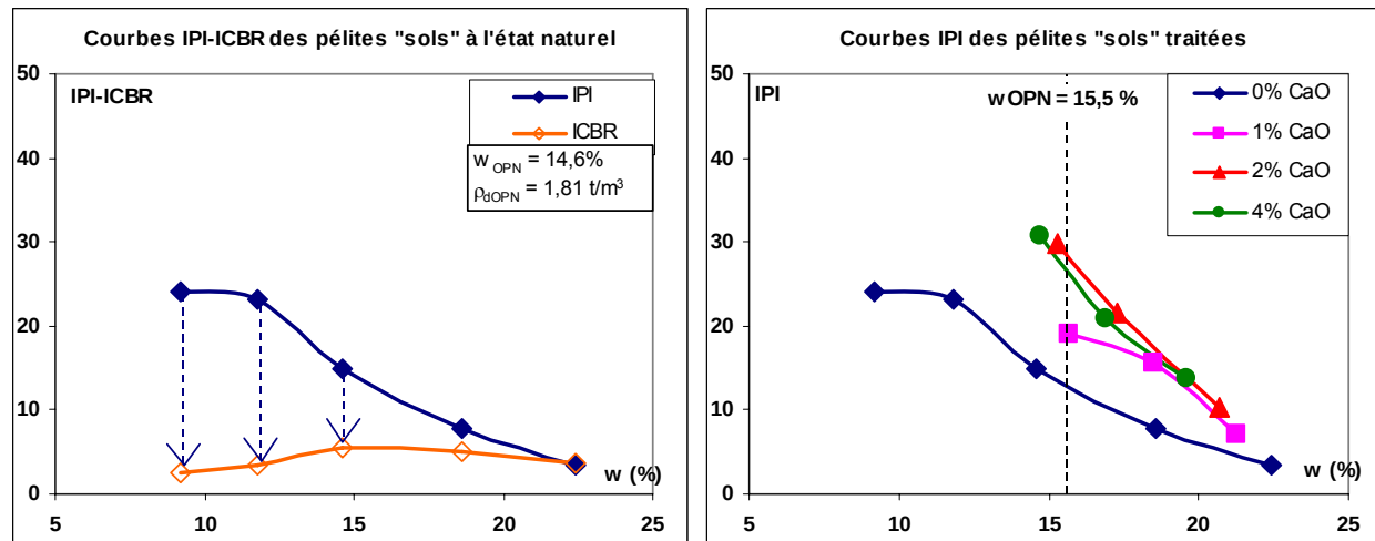
Figure 2 : courbes IPI et ICBR – immersion des pélites altérées à l'état naturel et traitées à la chaux. Références Proctor Normal du matériau traité à 1 % de chaux vive : w_{OPN} = 15,5\% , \rho_{dOPN} = 1,74 \text{ t/m}^3
