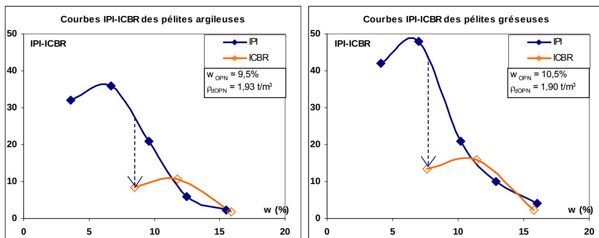
Figure 4 : courbes IPI et ICBR – immersion des pérites indurées réduites en fraction 0/25 mm
