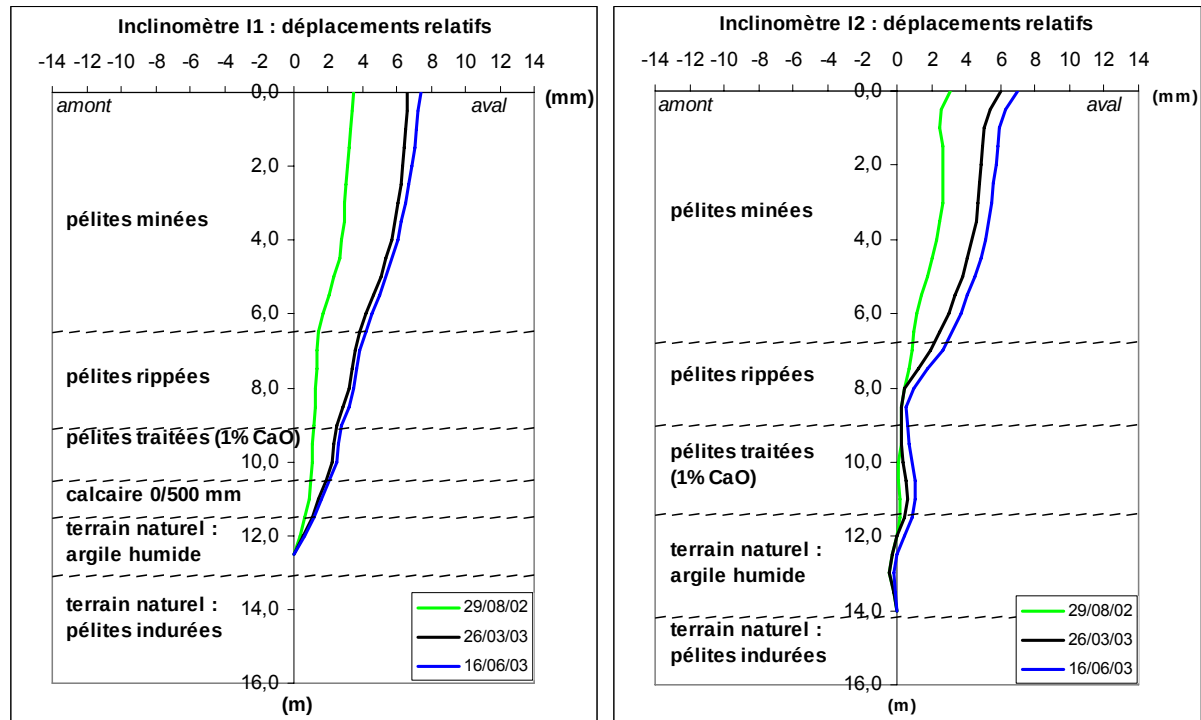
Figure 10 : mesures inclinométriques effectuées entre juin 2002 et juin 2003
