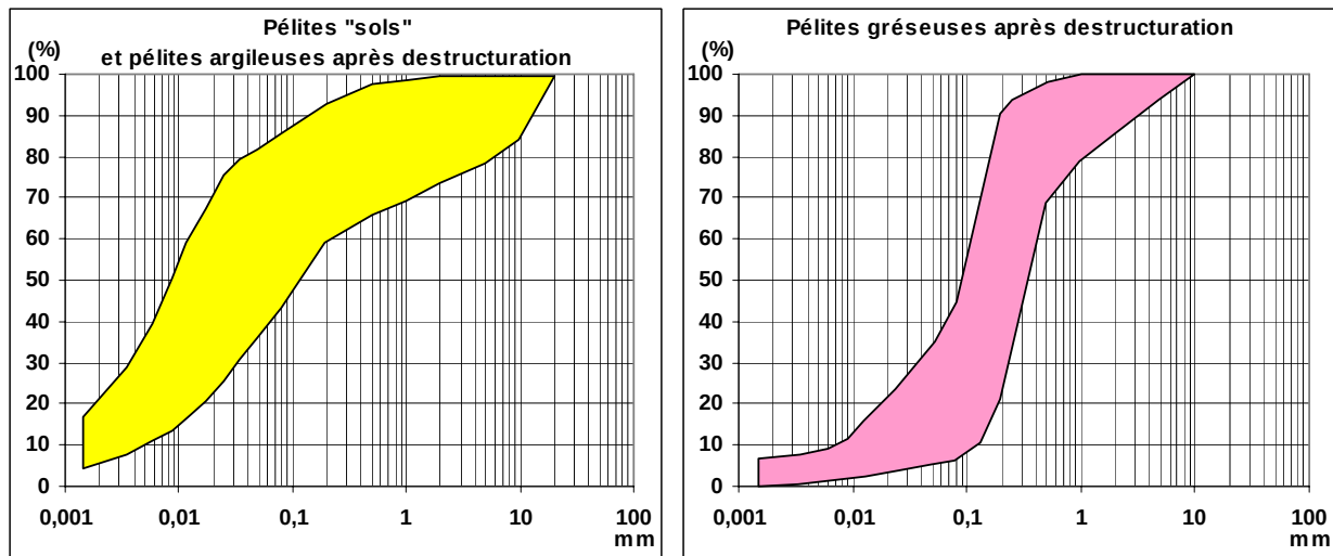
Figure 1 : fuseau granulométrique des pélites rocheuses destructurées après l'essai de dégradabilité
