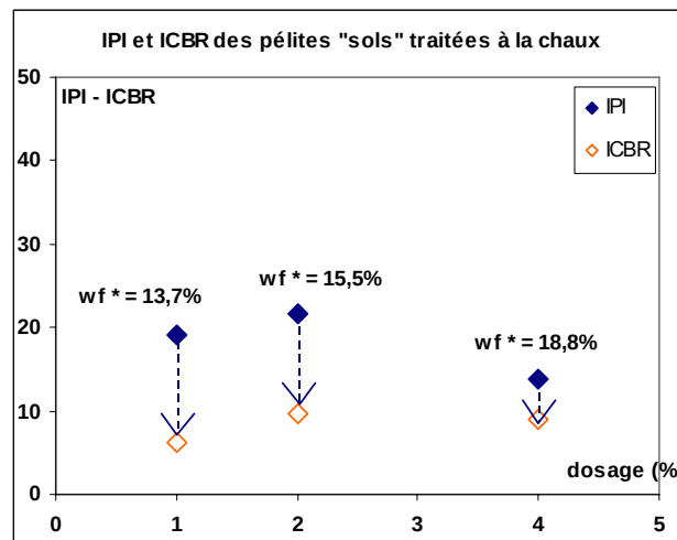
Figure 3 : IPI et ICBR-immersion sur le matériau traité * wf : teneur en eau après traitement
