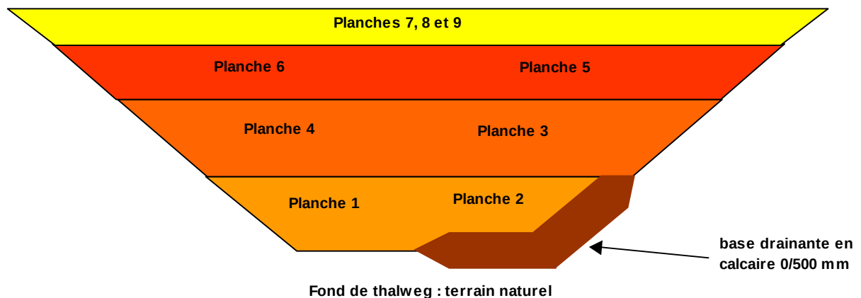
Figure 7 : profil en long schématique de la disposition des planches d'essai
